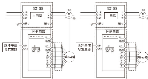
使用变频器内部电源接线图
