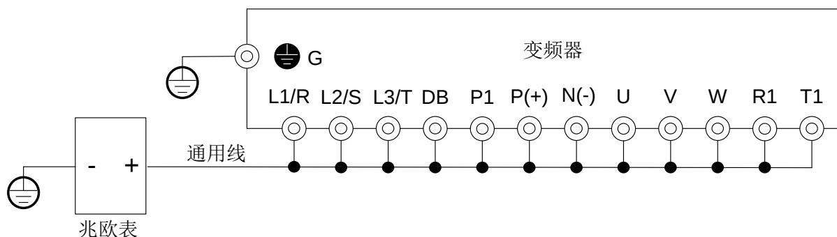
图 8.2 主回路绝缘电阻测试接线图
