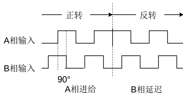
90 度相位差 A, B 相
