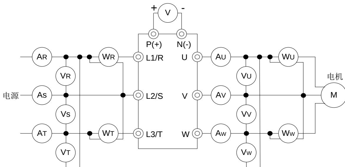
图 8.1 仪表的接线图
