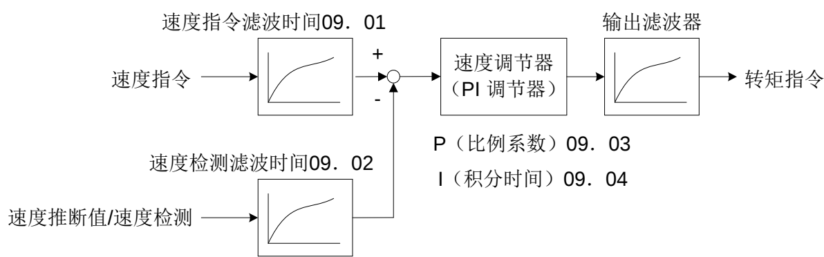
速度控制系统程序流程图
