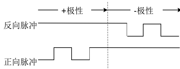
正向脉冲/反向脉冲
