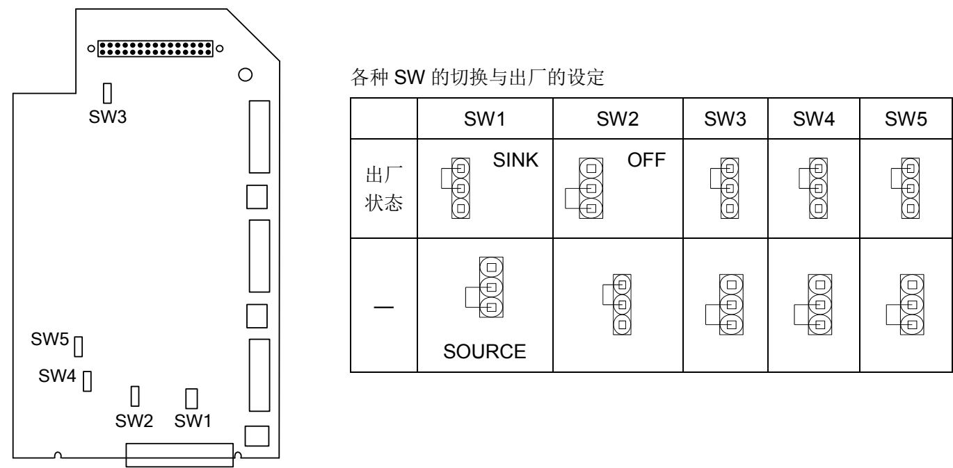
控制电路板上的各种开关的位置
