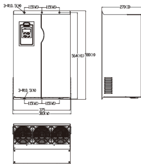
图D(S5100-4T37G~4T55G)
