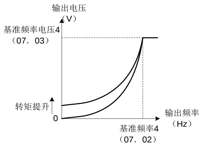
2 次幂降转矩特性 (07. 13 = 0)
