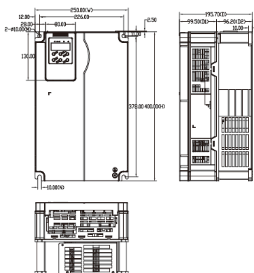
图B(S5100-4T15G~4T22G)
