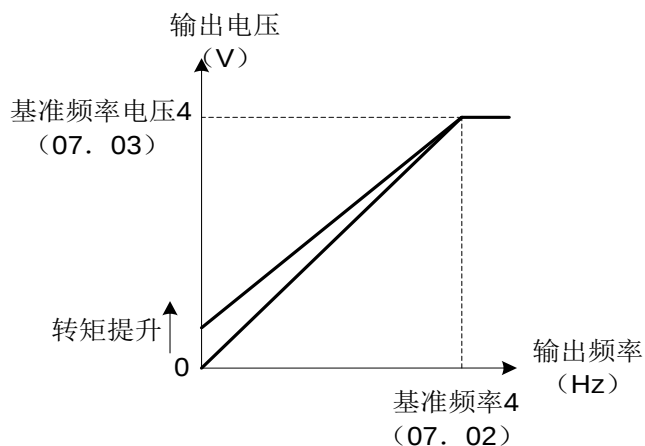
直线 V/f 特性 (07. 13 = 1)
