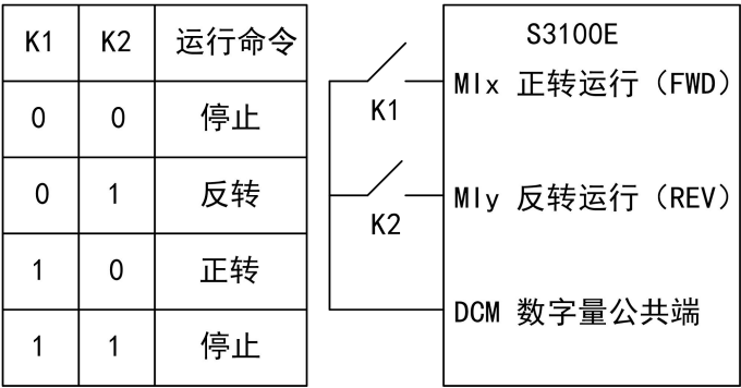
图 5-6 两线式模式 1
