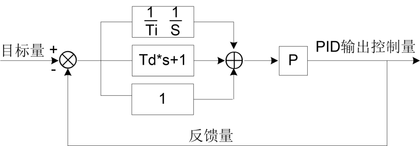
图 5-25 过程 PID 原理框图
